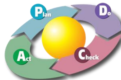
Figuur 1. PDCA-cyclus
